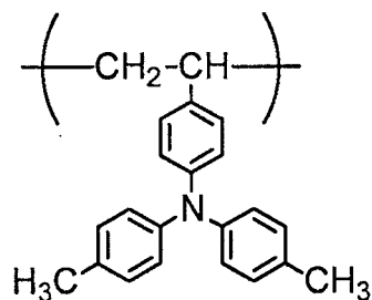
[化学式 21]
