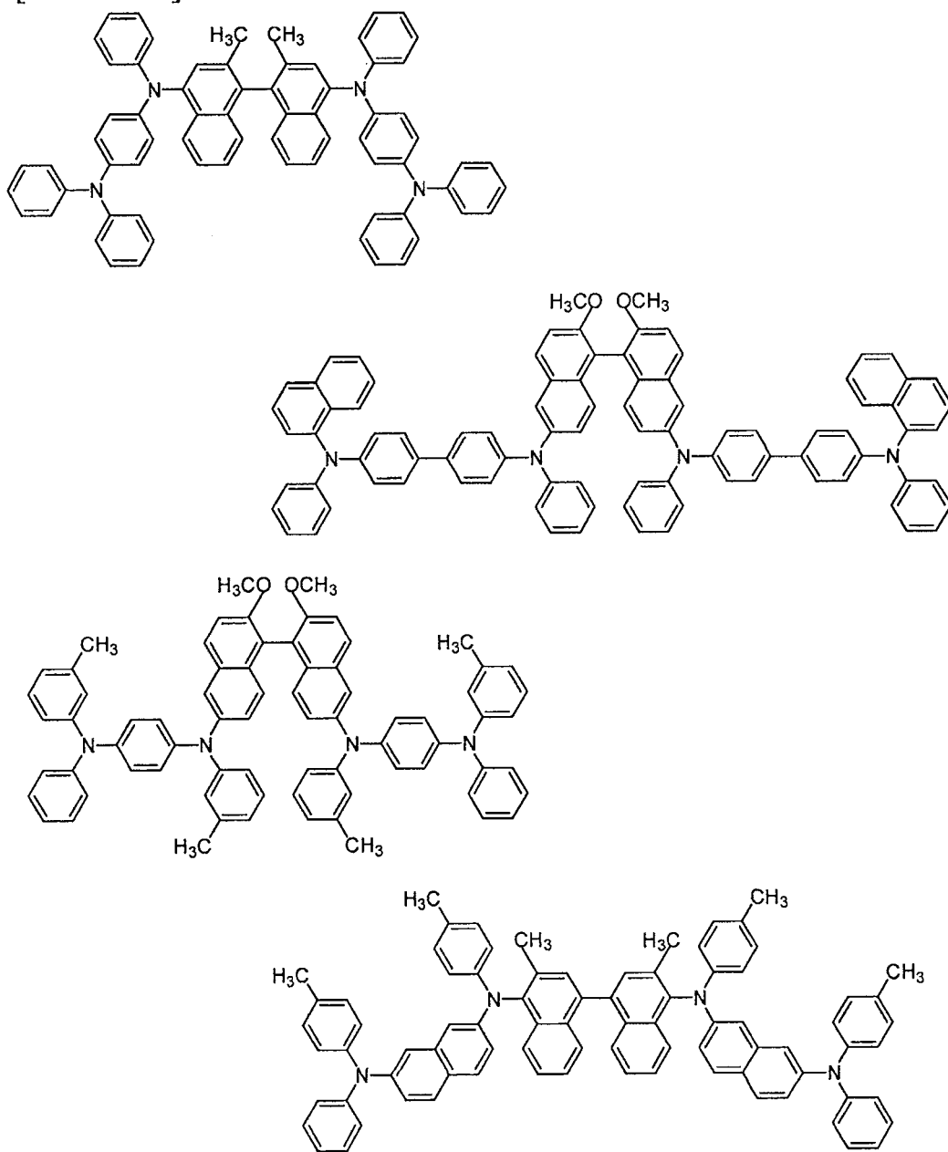
[化学式 23]
