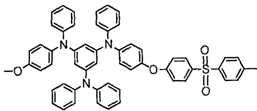
[化学式 17]
