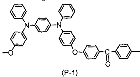
[化学式 14]
