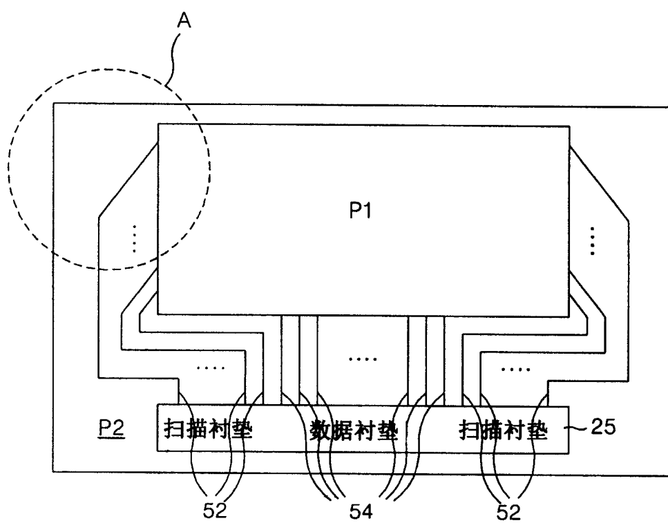
图1 现有技术
