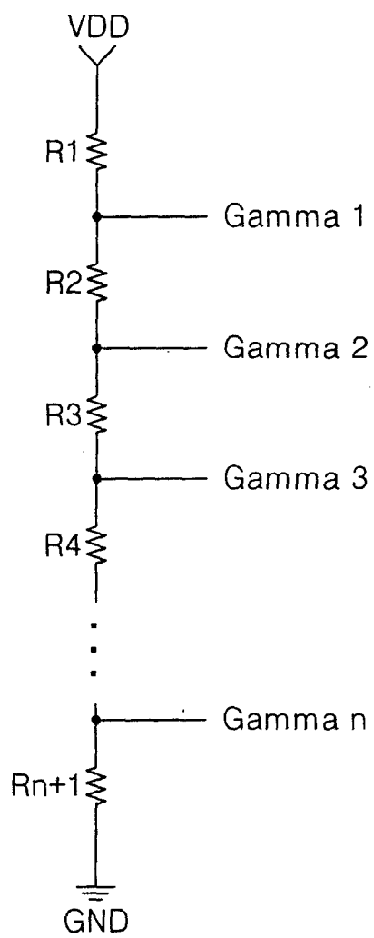
图 4 现有技术
