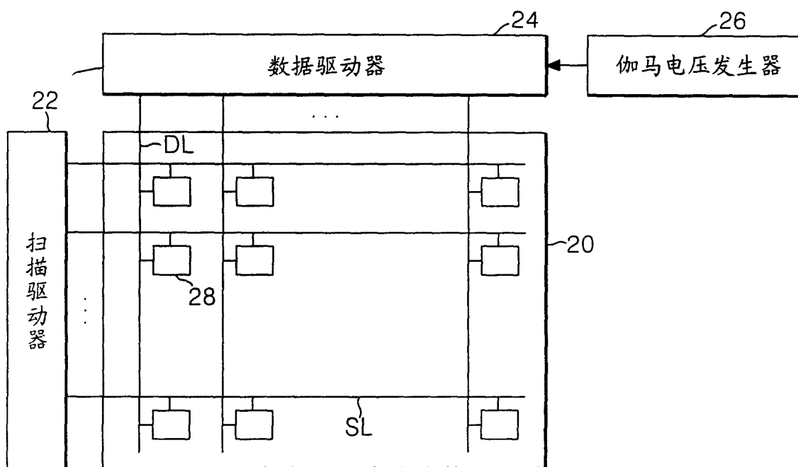
图 1 现有技术
