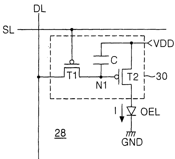
图 2 现有技术
