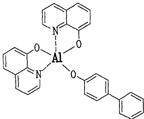
BAlq3
