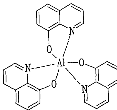
Alq3
