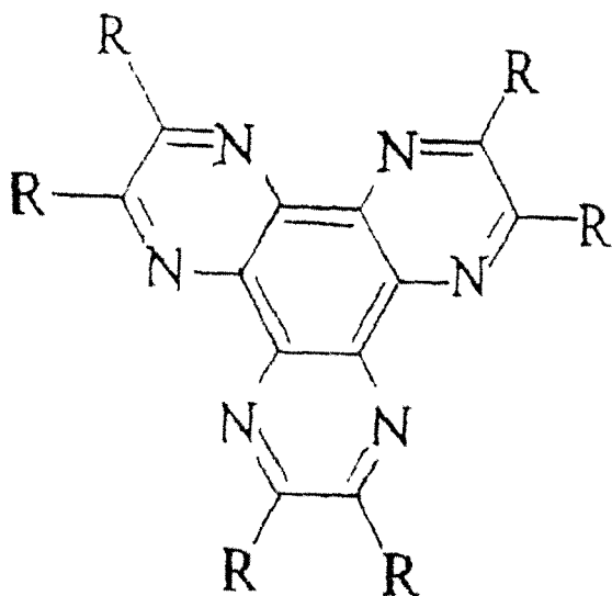
[结构式 2]
