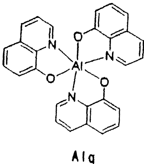
[结构式 12]
