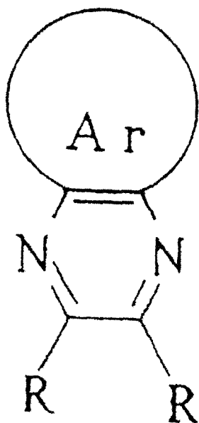
[结构式 1]
