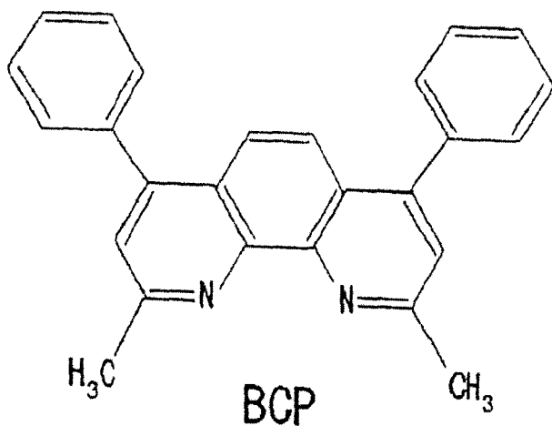
[结构式 13]
