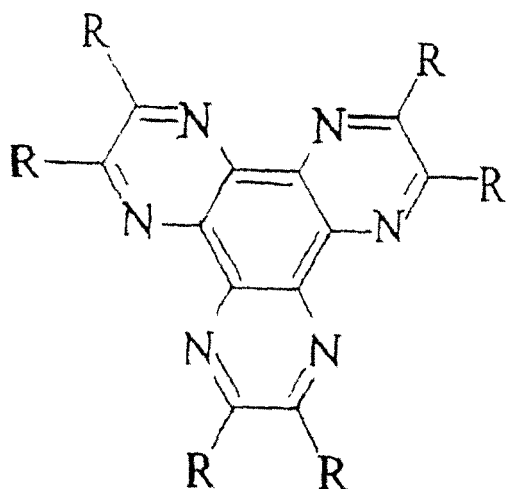
[结构式 2]
