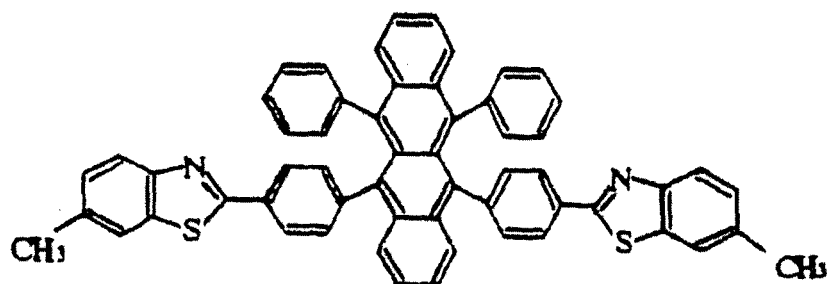
[结构式 10]
