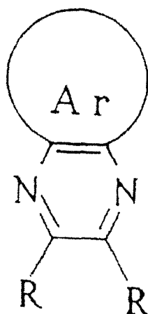
[结构式 1]
