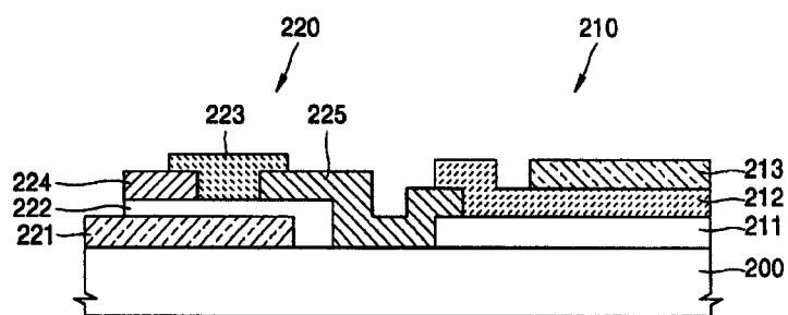
图 3 (现有技术)
