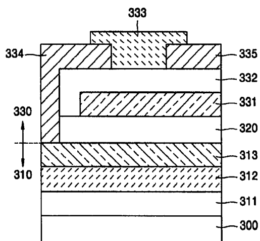
图 4 (现有技术)
