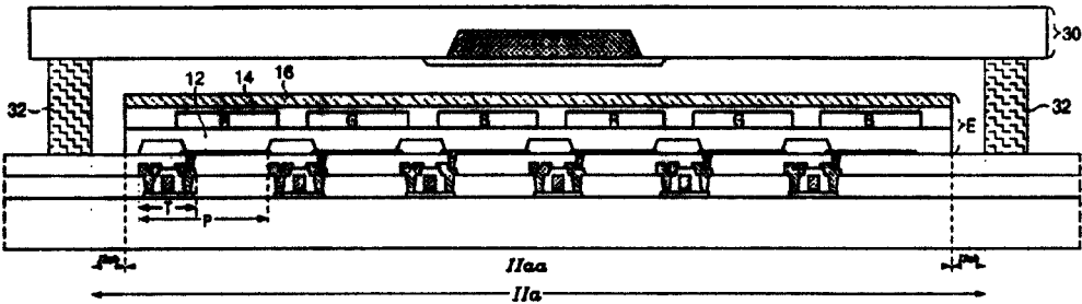
图 2B (现有技术)
