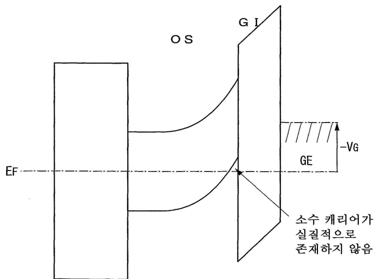
B-B' 단면의 에너지 밴드도 ( -V_G )
