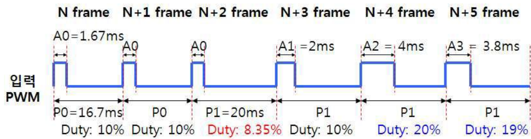
도면6
