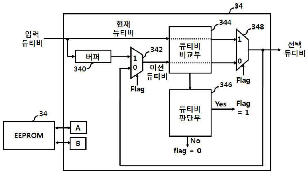
도면6
