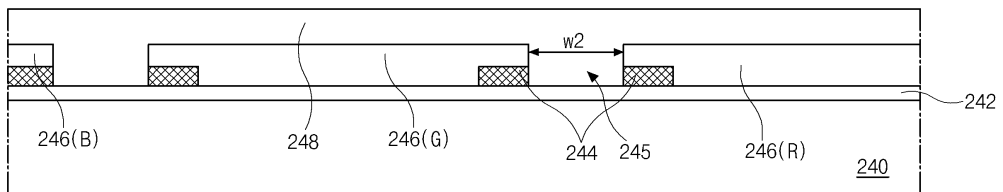
도면3e
