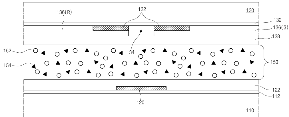
도면2b
