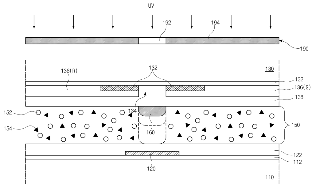
도면3a
