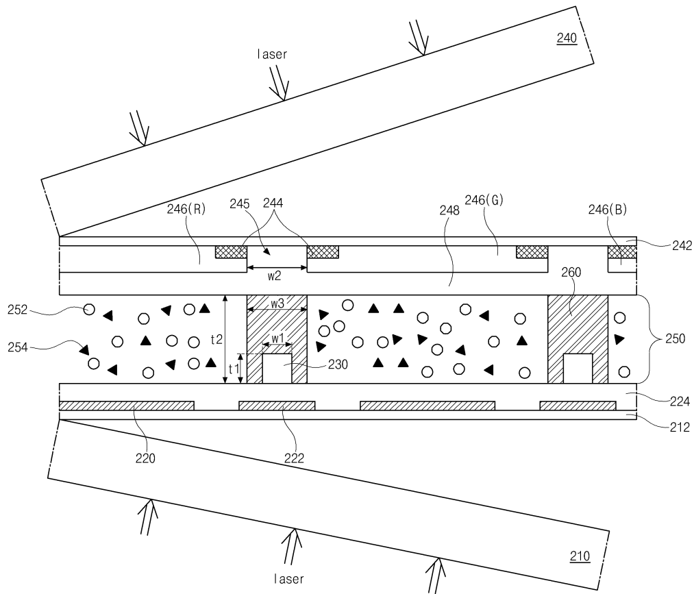
도면3g
