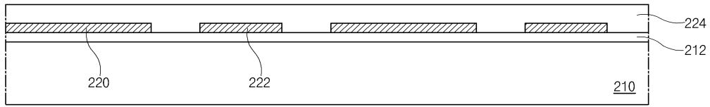
도면3c
