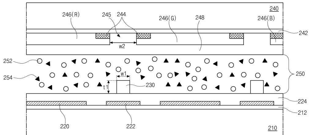
도면3e
