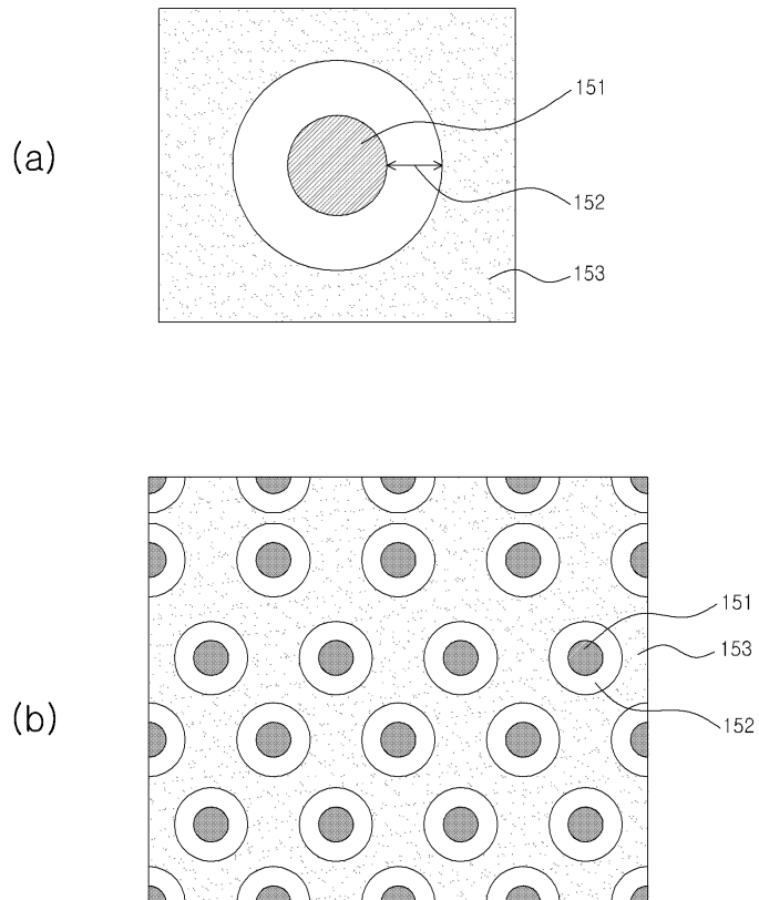
도면3b
