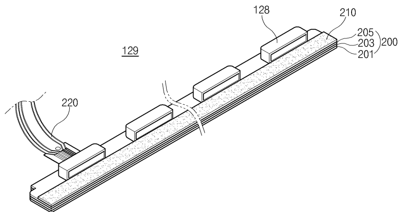
도면3b
