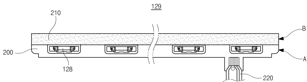
도면3b
