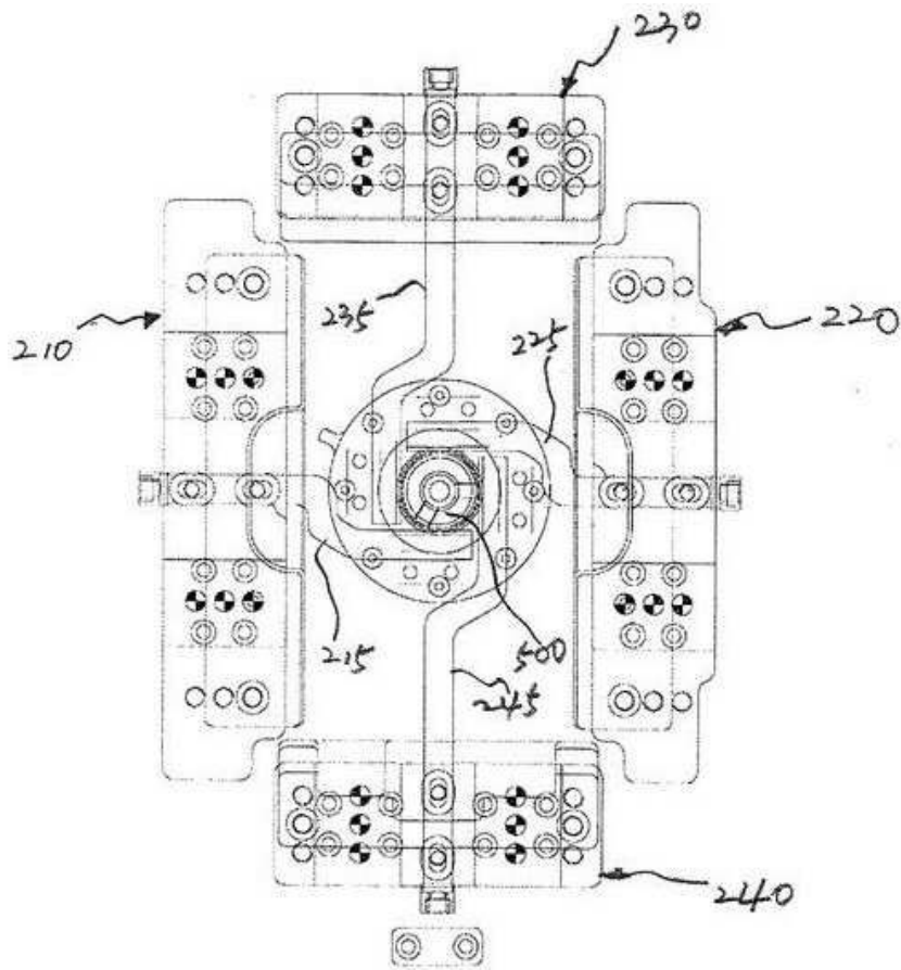
도면4a
