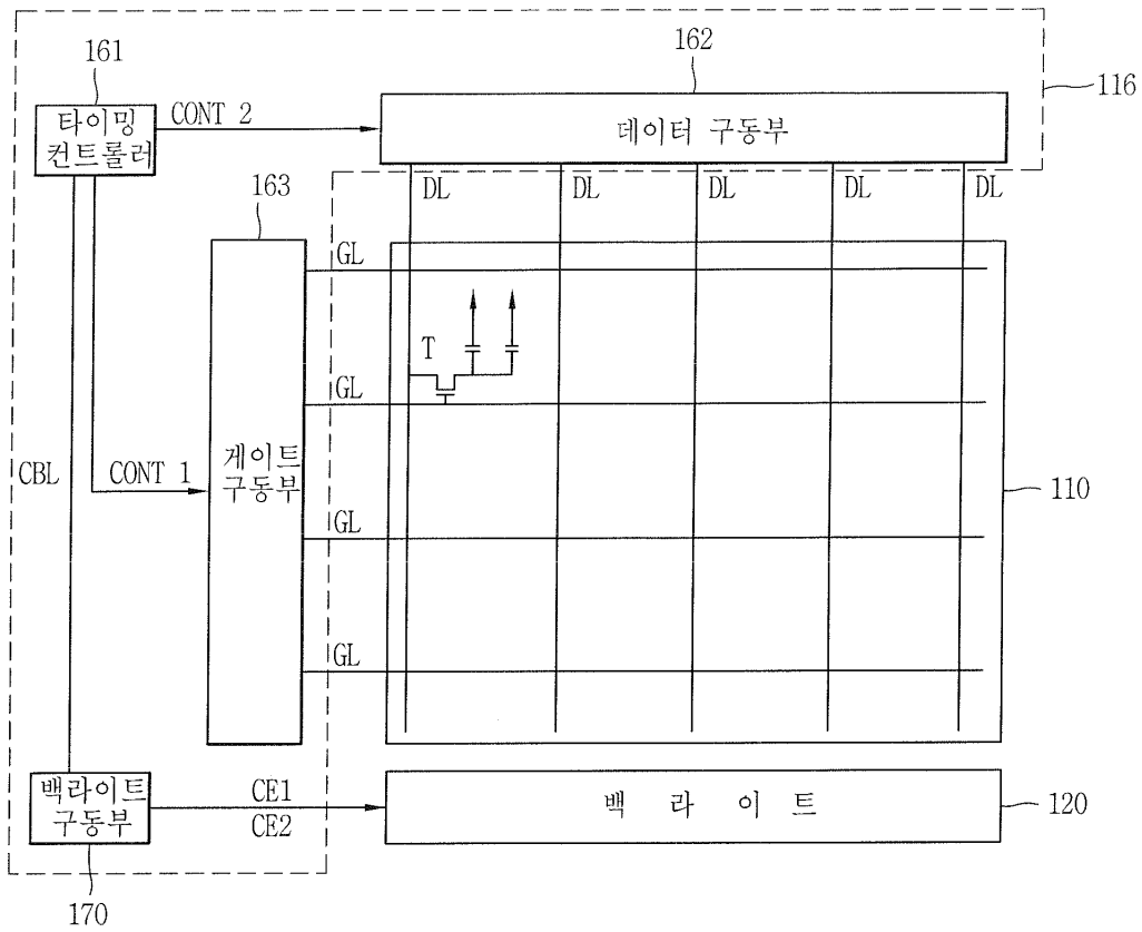
도면4a
