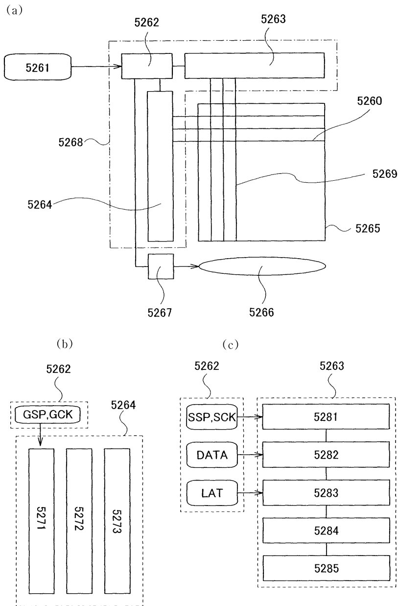
도면43
