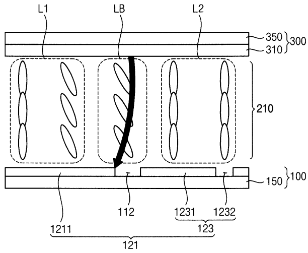
도면10b
