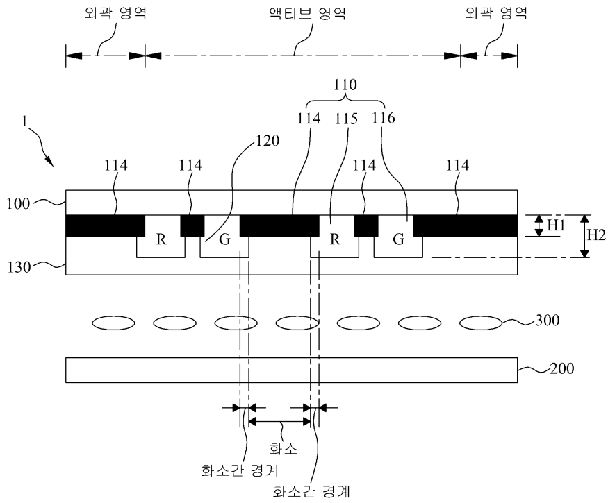
도면9
