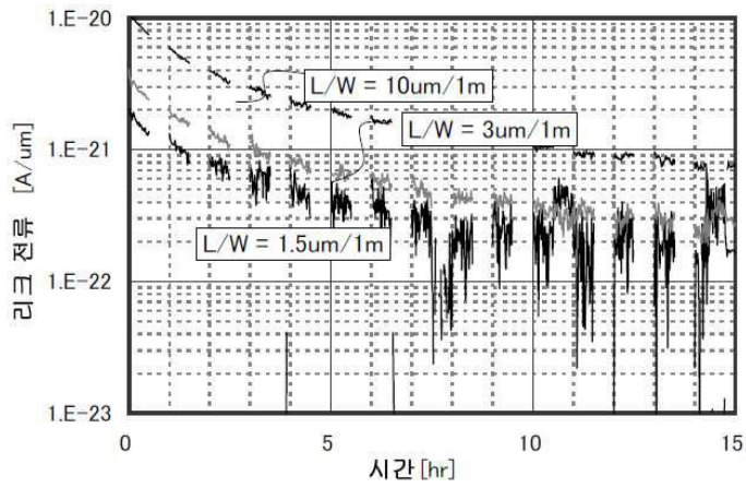
도면12
