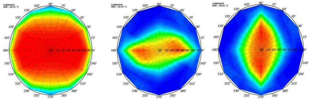
[a] 시야각제어유닛이 없는 상태의 White 휘도분포 [b] 시야각제어 유닛이 있는 상태의 White 휘도분포
