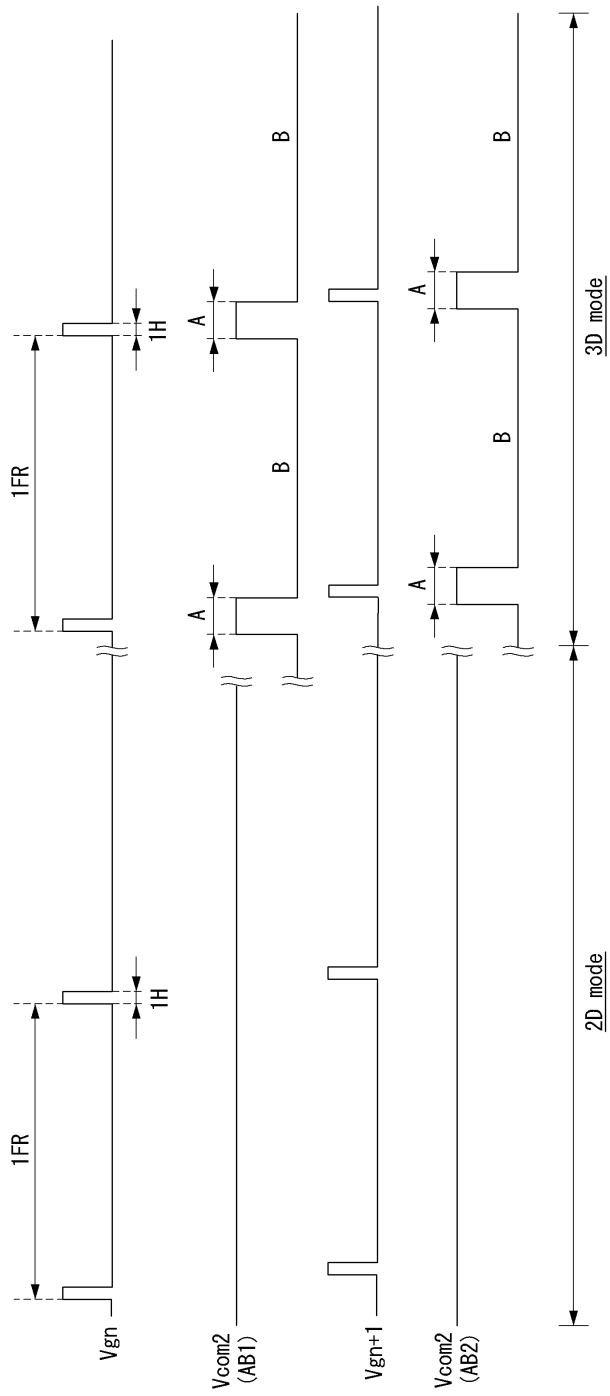
도면9
