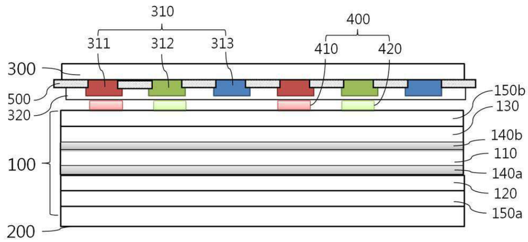
도면2
