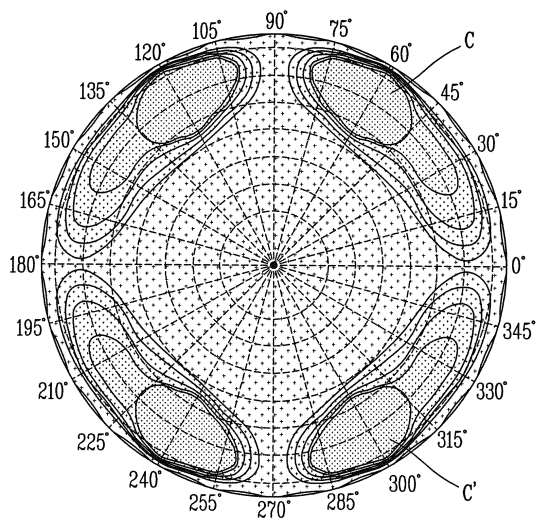
도면6b
