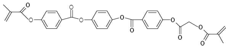
구조식 XVII-R4
