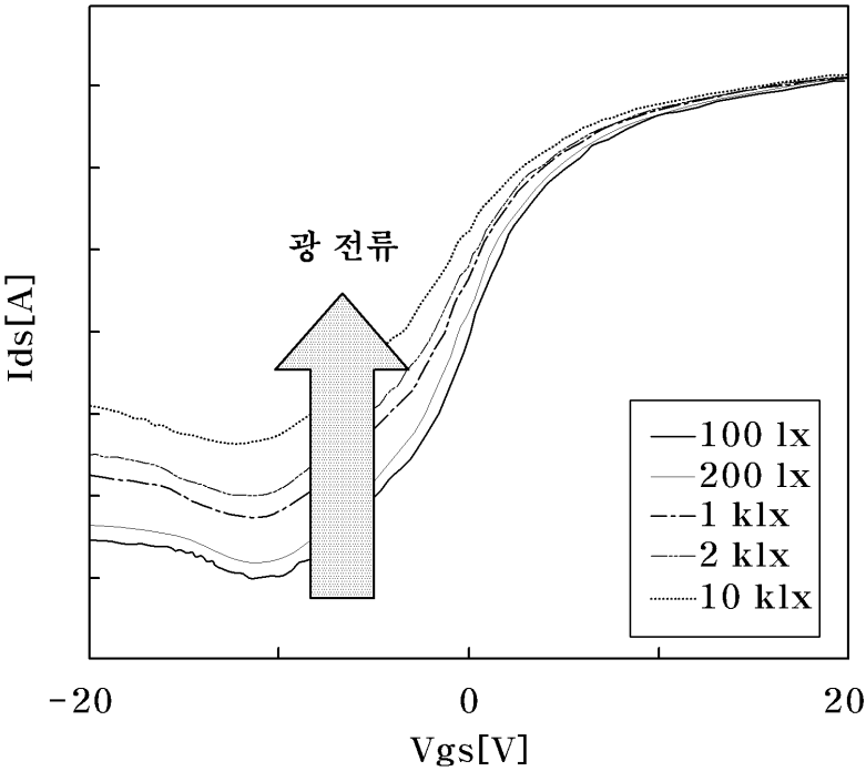
조도별 Transfer Curve(V ds =5V)
