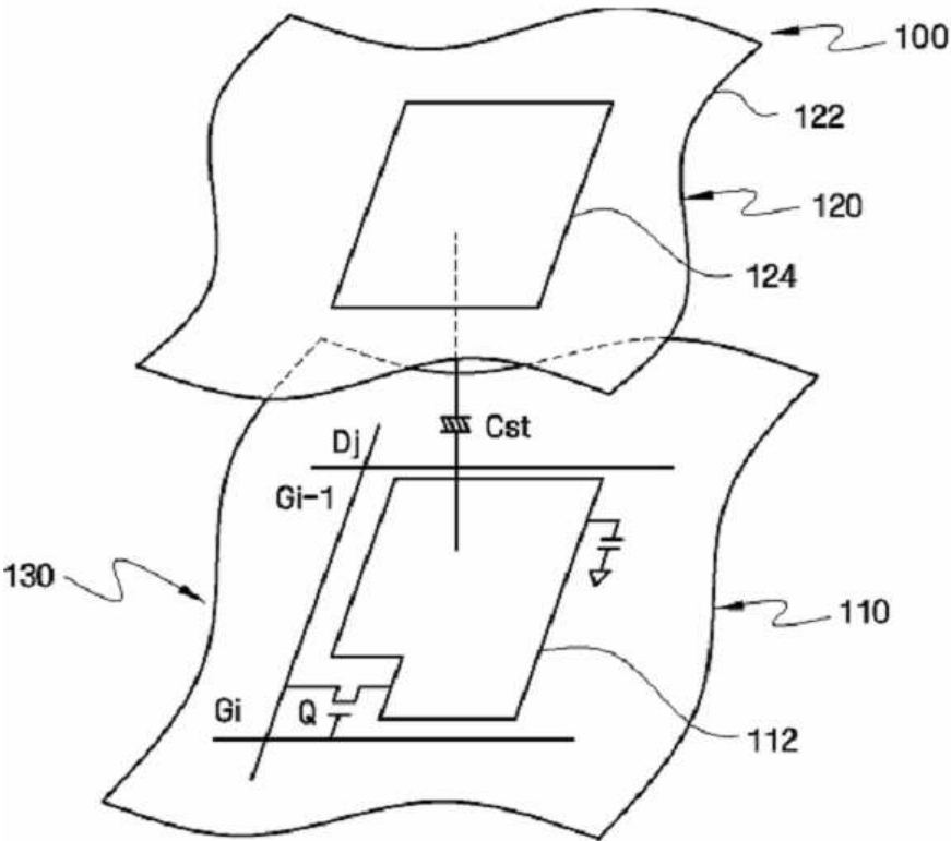
도면4a
