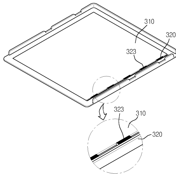
도면5
