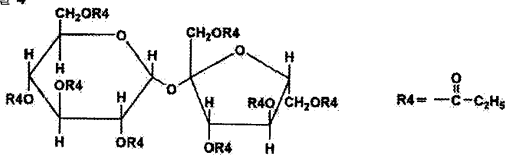
화합물 4
