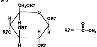
화합물 8
