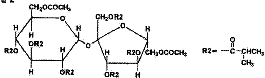
화합물 3
