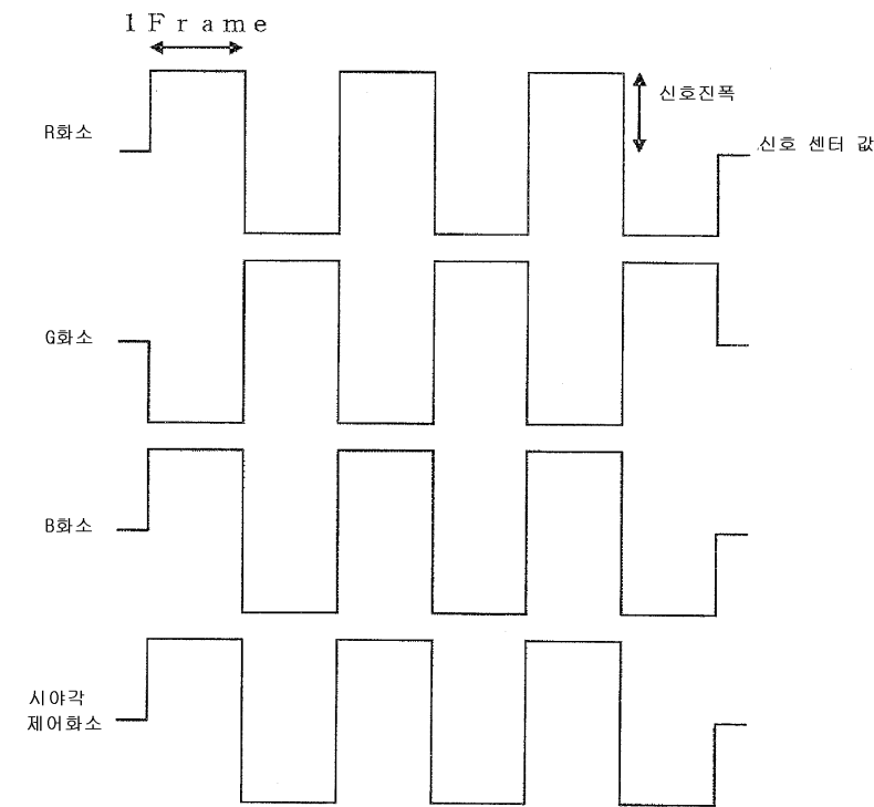
DOT 반전의 신호라인 파형
