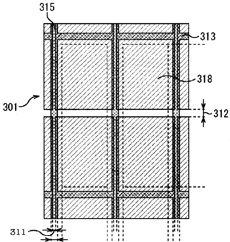
화소전극의 어느 기판측에서의 광학마스크의 배치
