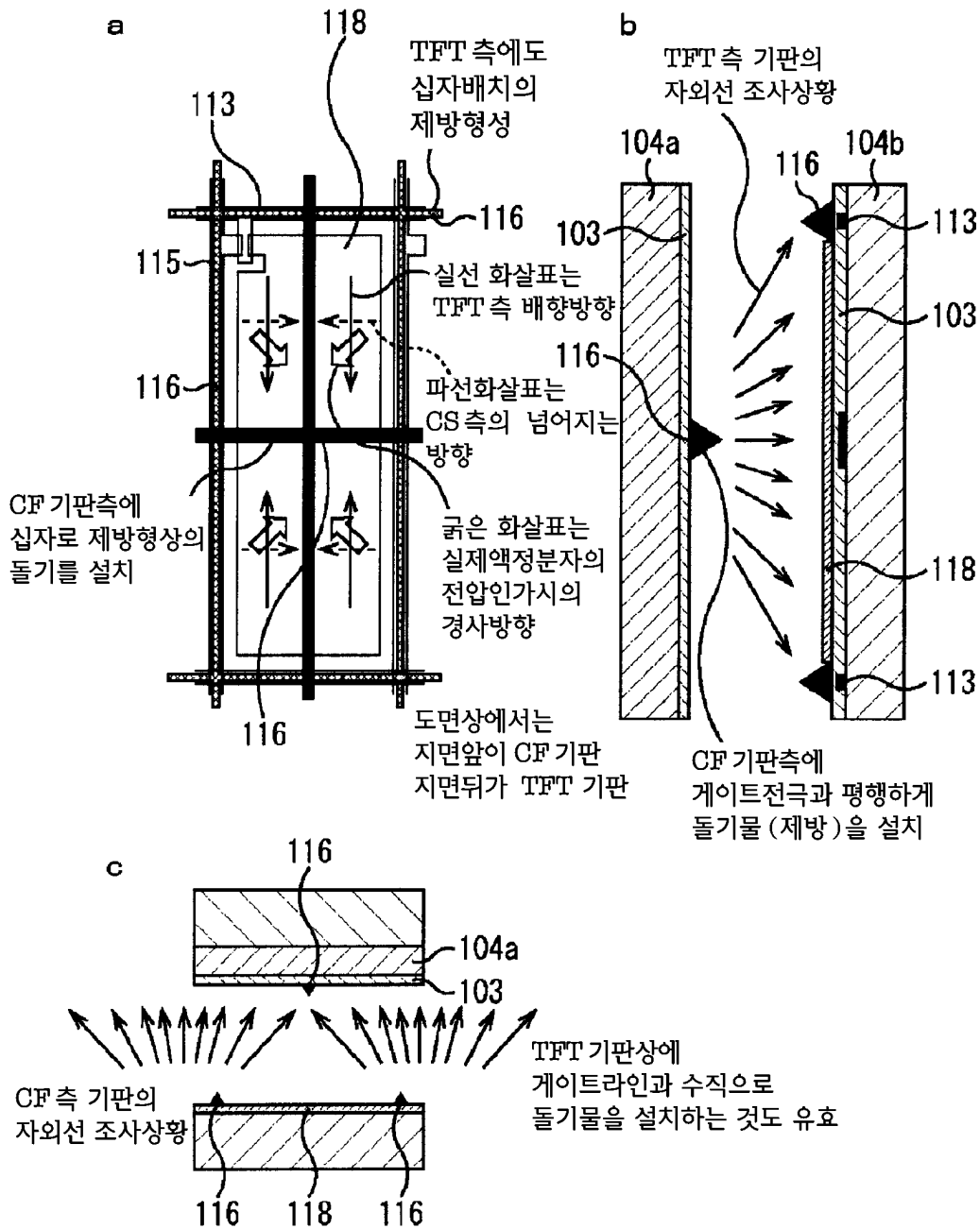
4 분할 배향을 실현함에 있어서의 자외선 조사방법 예
