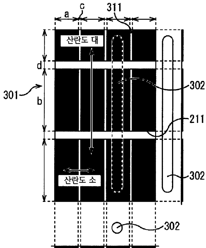
램프의 산란성과 광학마스크의 슬릿의 배치관계
