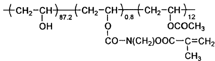
일반식 (4)
