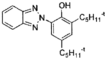
구조식 (M-2)
