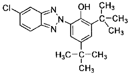
구조식 (M-1)
