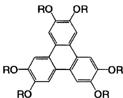
일반식 (D-1)
