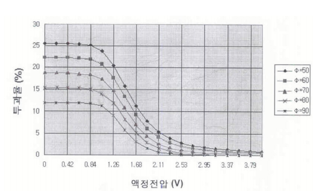
도면 2
