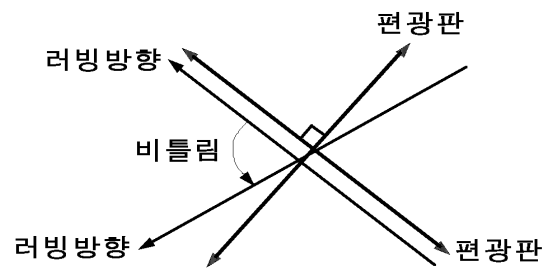
도면 3
