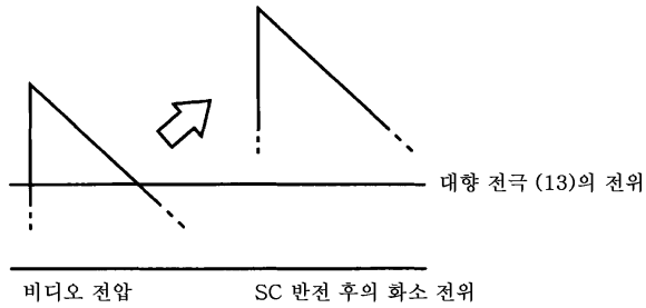
(b) 화소 전위 (화소 GS12)
