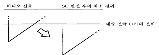
(a) 화소 전위 (화소 GS11)
