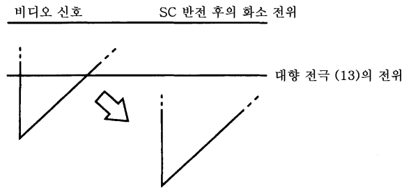
(a) 화소 전위 (화소 GS11)
