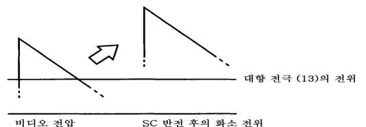
(b) 화소 전위 (화소 GS12)
