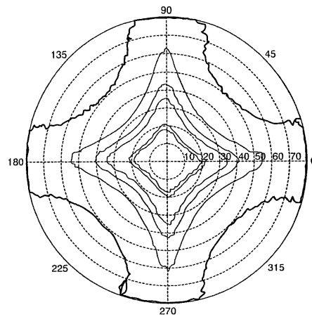
비교예 2의 등콘트라스트 곡선
