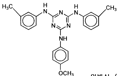
일반식 (12)
