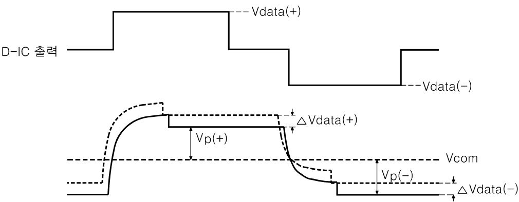
패널위치 'B'에서 V_{com} 을 최적화 한 경우
