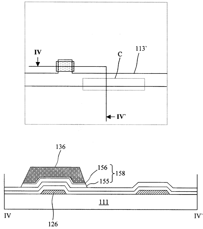
도면4b
