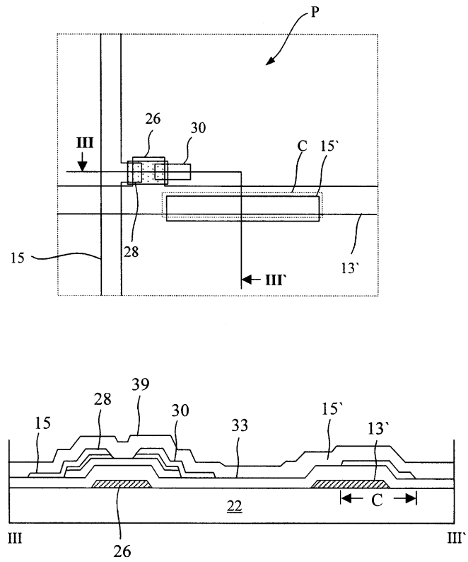
도면3d
