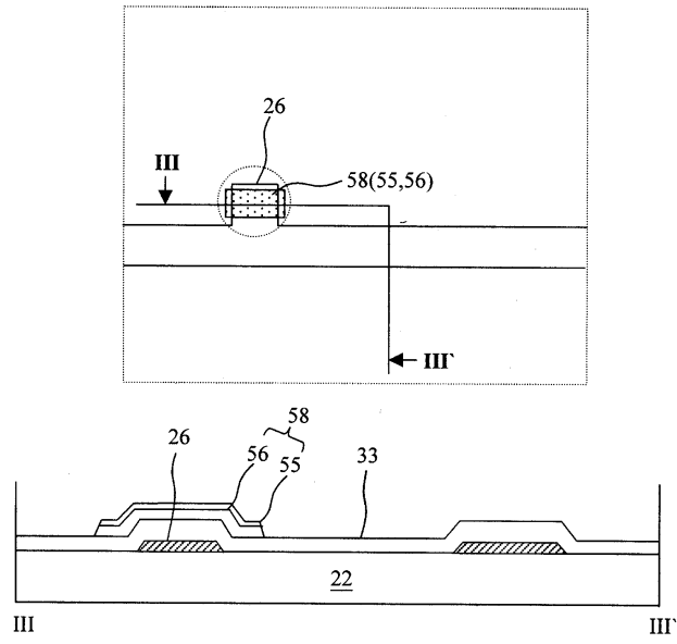
도면3d
