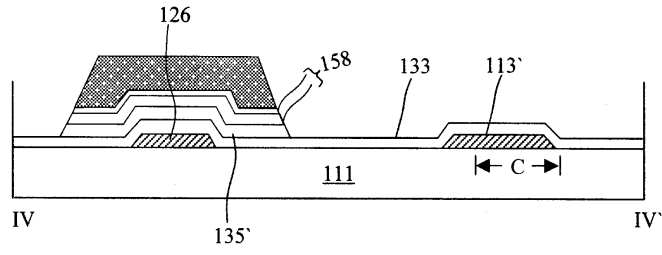
도면4d
