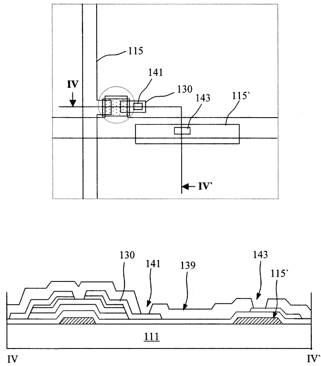
도면4f
