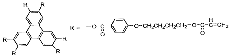
디스코틱 액정성분자 (1)
