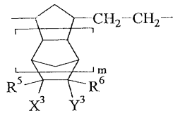
일반식 (III)
