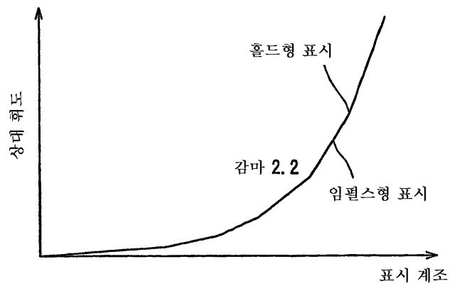
액정 표시 장치의 감마 특성
