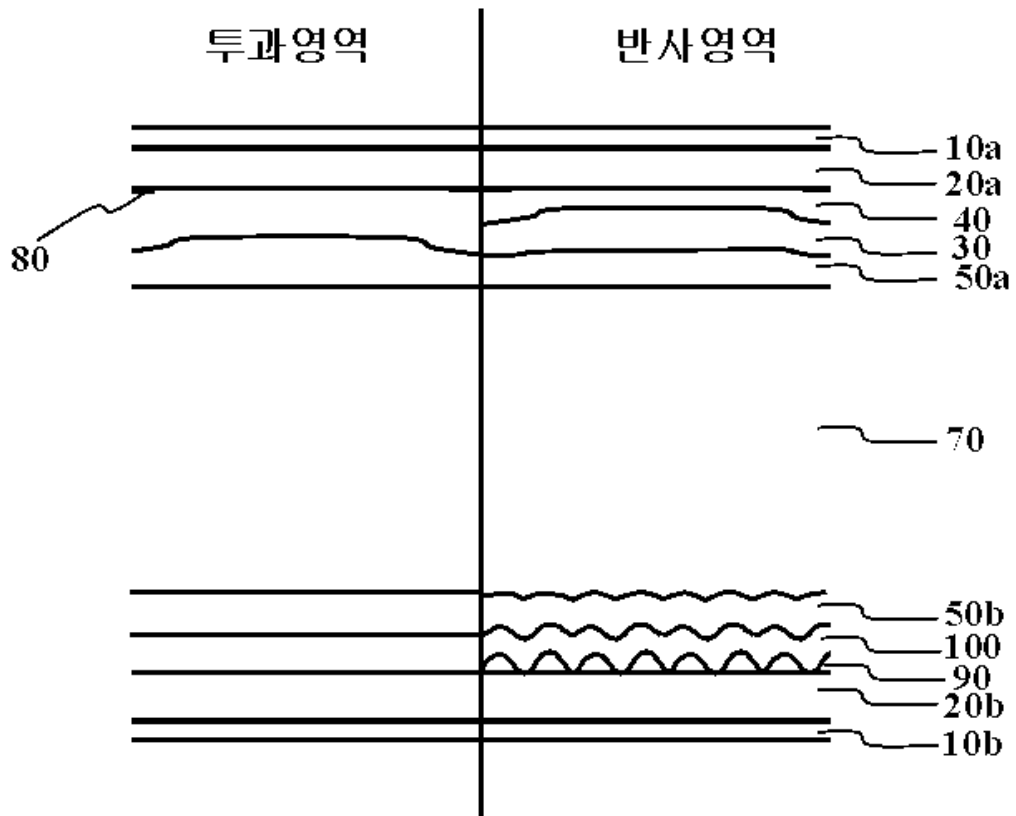
도면5a
