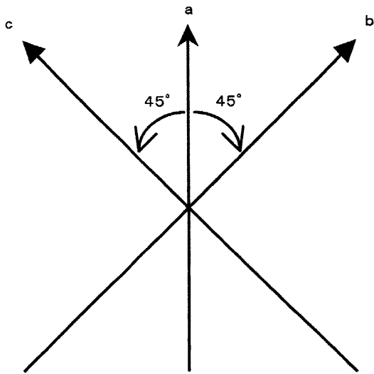
a: 배향 제어용의 돌기(29)의 장축 방향 b: 편광판(32a)의 흡수축 c: 편광판(32b)의 흡수축
