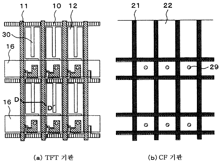
(a) TFT 기판 (b) CF 기판
