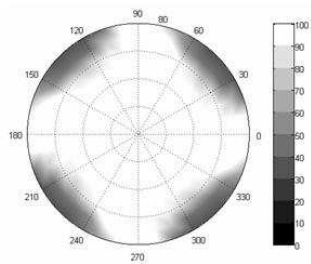
실시에5의 시야각 특성
