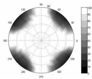
실시에1의 시야각 특성
