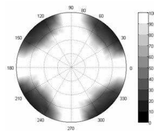
실시에2의 시야각 특성
