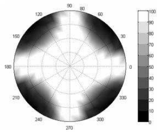
실시에3의 시야각 특성
