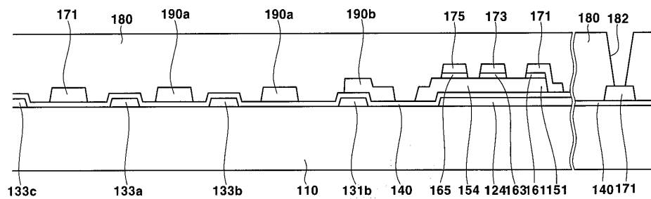
도면21
