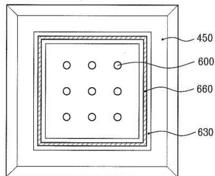
도면6a
