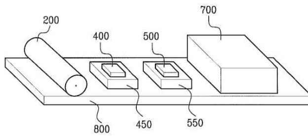
도면6a
