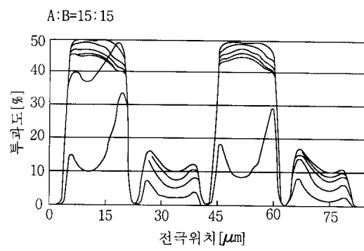
도면4a
