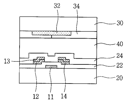
도면2a
