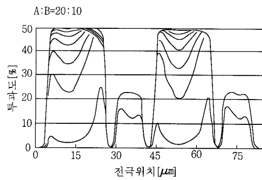
도면4c
