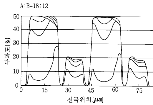
도면4b
