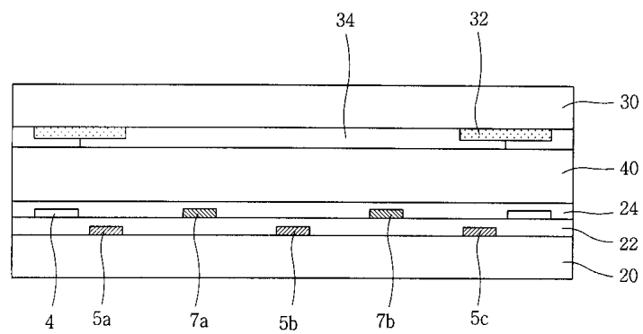
도면2b
