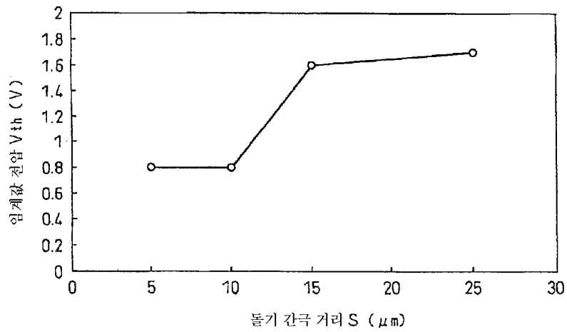
돌기 간극에 따른 임계값 전압의 변화
