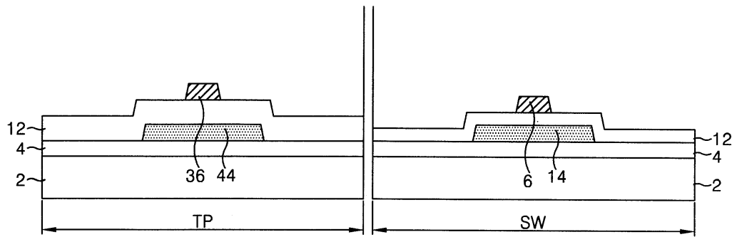
도면2d
