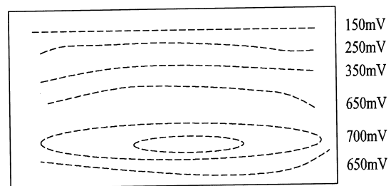
<기존 : Vcom 변동 측정 결과>
