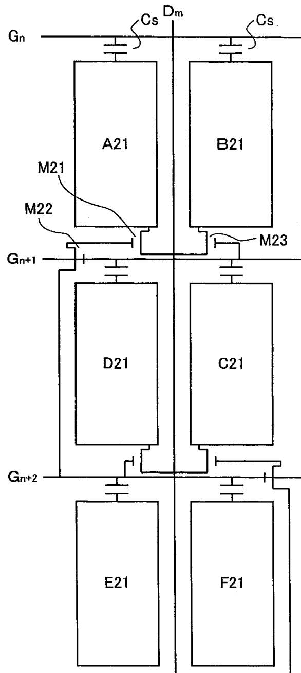
도면9
