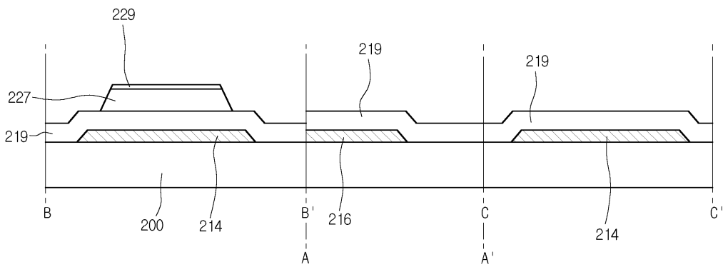
도면4b
