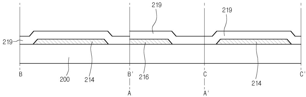
도면4a
