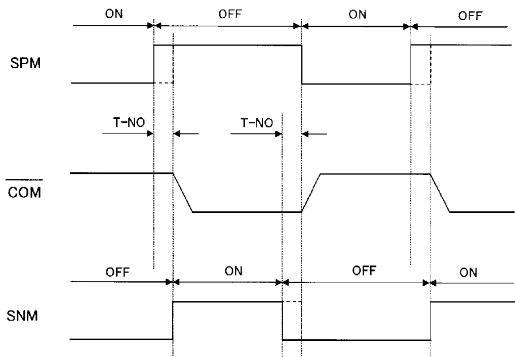
FIG. 7C
